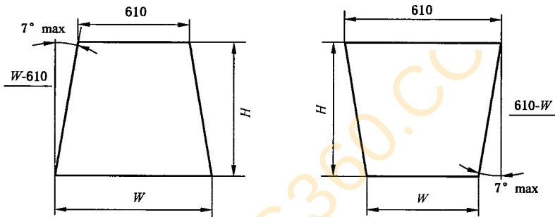
图 H.3 边截面风道管段
