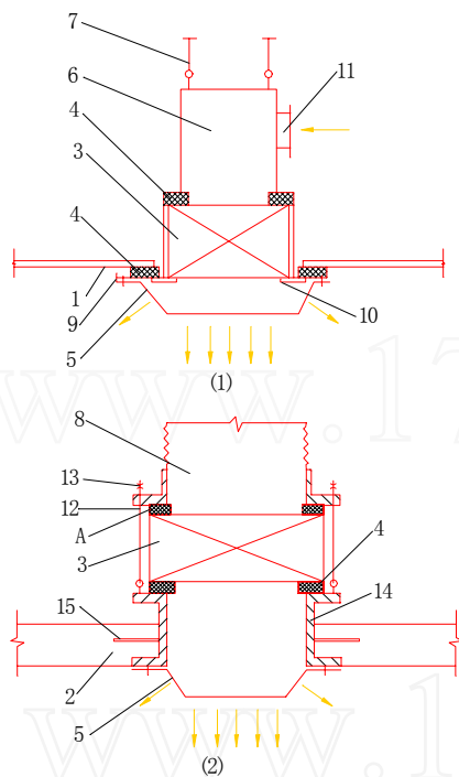
图 3.3.10 高效过滤器送风口安装示意图
