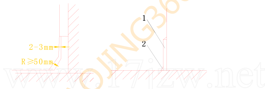
图 2.3.8 踢脚板部分做法 1—踢脚板; 2—密封嵌固材料
