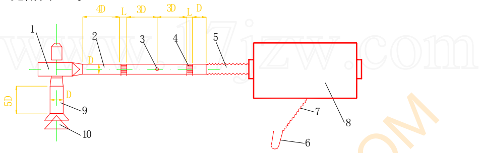
附图 4-1 空调器漏风率检测装置
