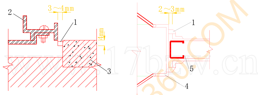
图 2.3.2 缝隙密封宽度
