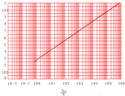
附图 6-3 乱流洁净室自净时间算图
